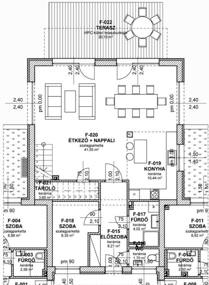
földszinti alaprajz
