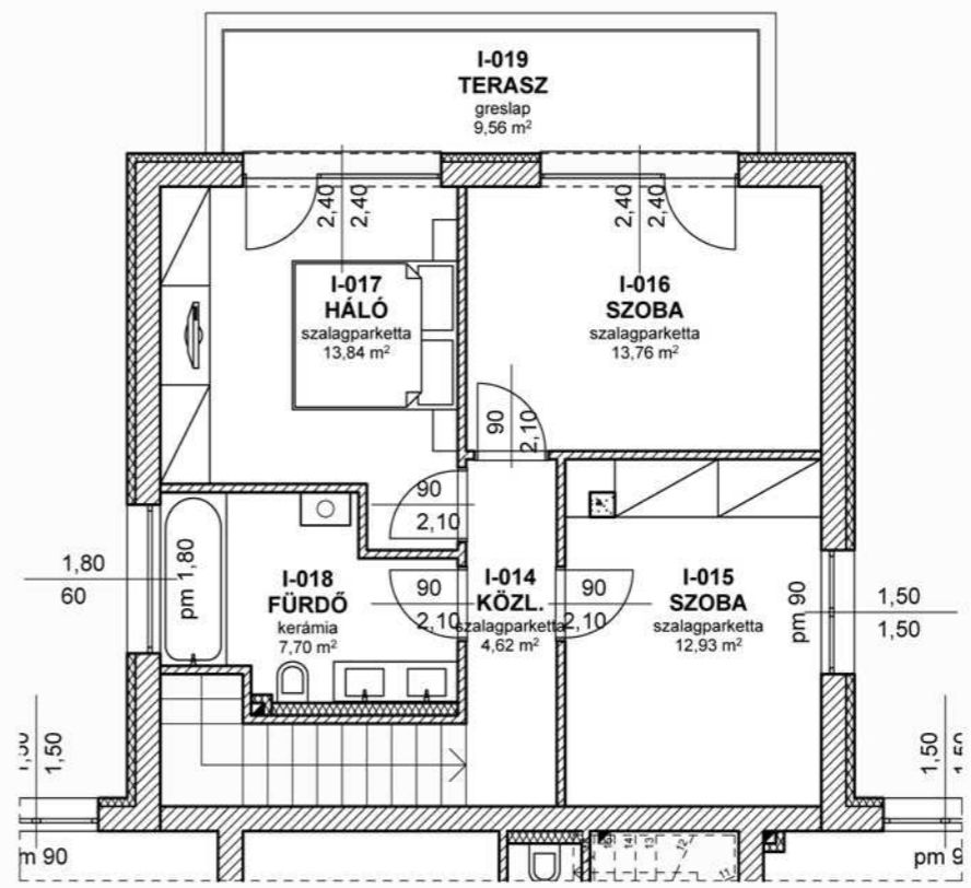
I. emeleti alaprajz
