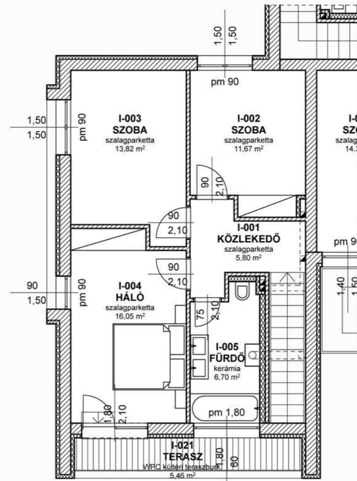
I. emeleti alaprajz
