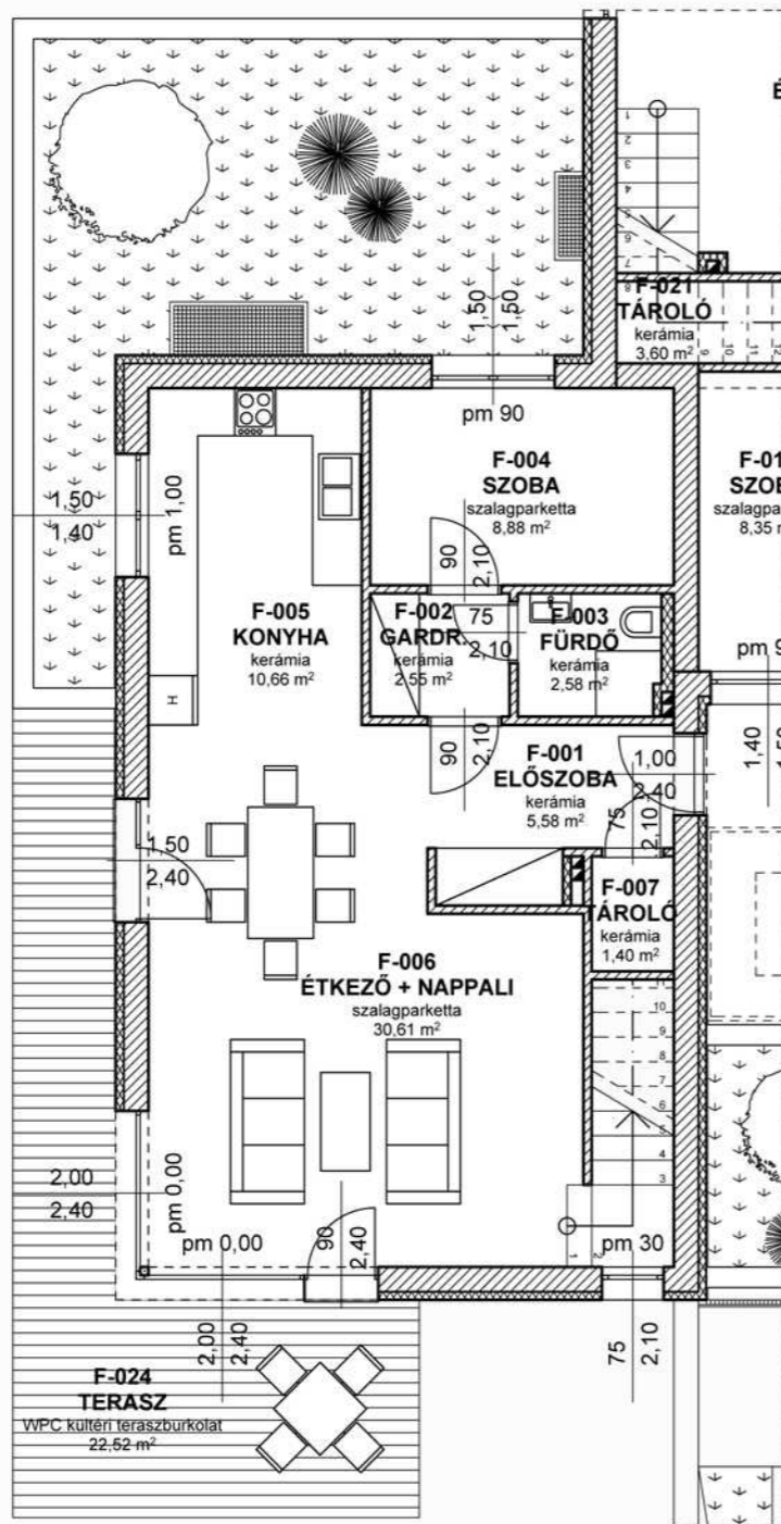
földszinti alaprajz
